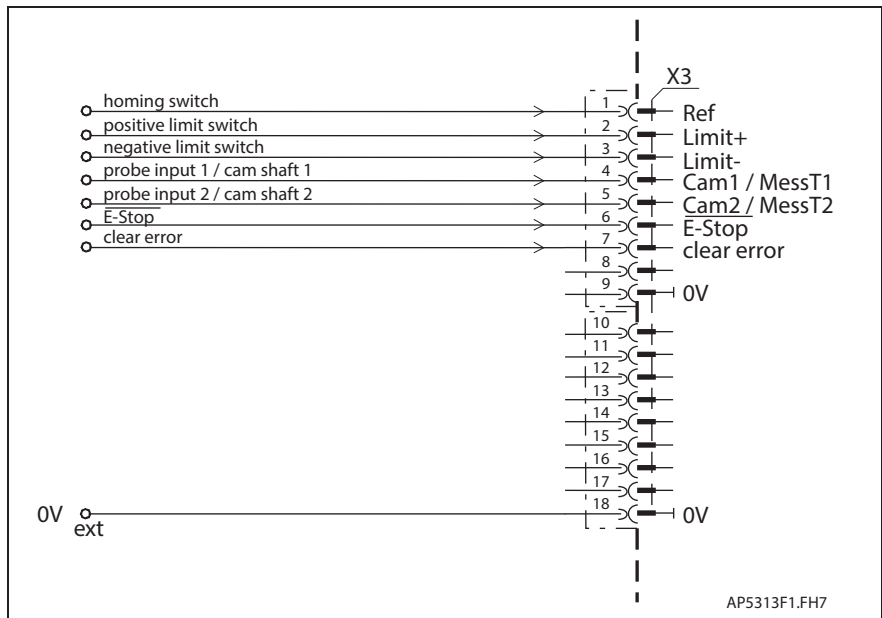
Fig. 4-66: Digital inputs
