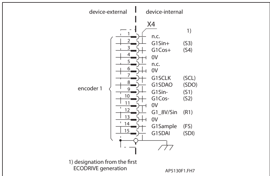
Fig. 4-84: Encoder 1
