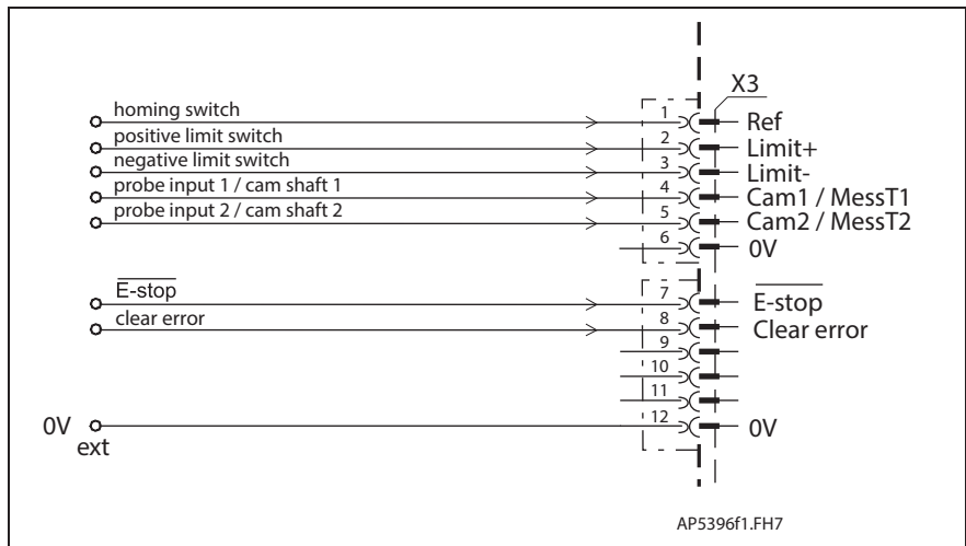
Fig. 5-38: Digital inputs
