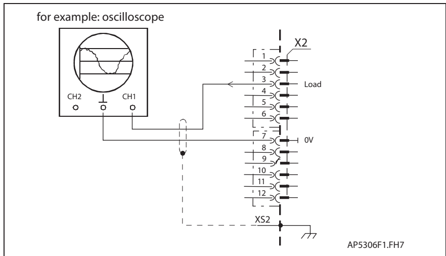
Fig. 6-26: Output load
